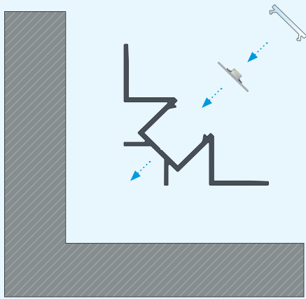
PL Instrukcja montażu profilu VIGO z kloszem BASIC.
