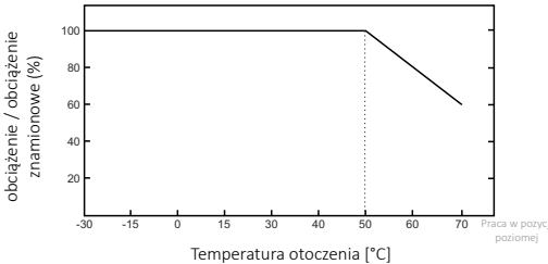
CHARAKTERYSTYKA OBCIĄŻALNOŚCI W ZALEŻNOŚCI OD TEMPERATURY OTOCZENIA 230AC
